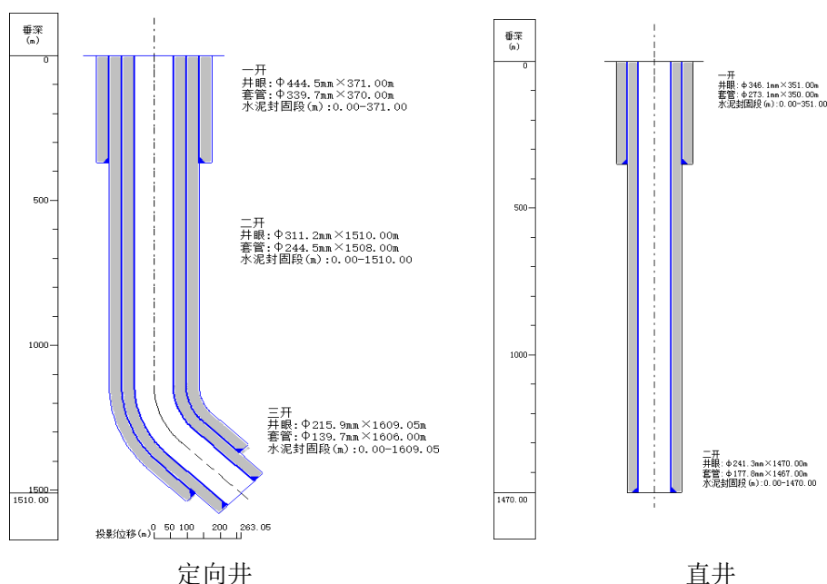
图 3-1 井身结构示意图
