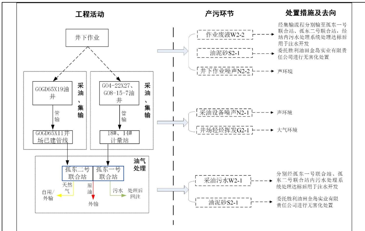
图 3-3 运营期主要工艺流程及产污环节
