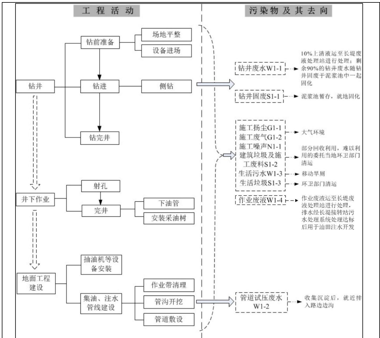
图 3-2 施工期主要工艺流程及产污环节
